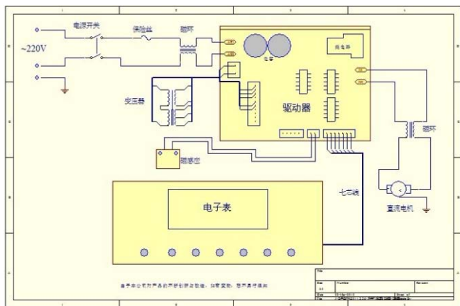
电路图
